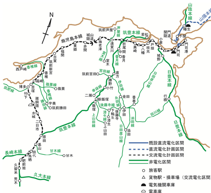
図1 国鉄北九州地区の路線と電化計画(昭和35年頃、貨物線・貨物支線を除く)
